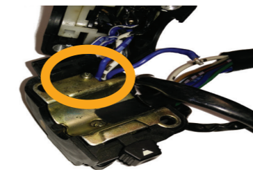
Abgedeckter Blinkerschalter
